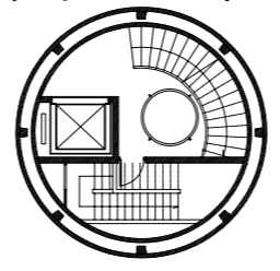
Plan du rez de chaussée N0
