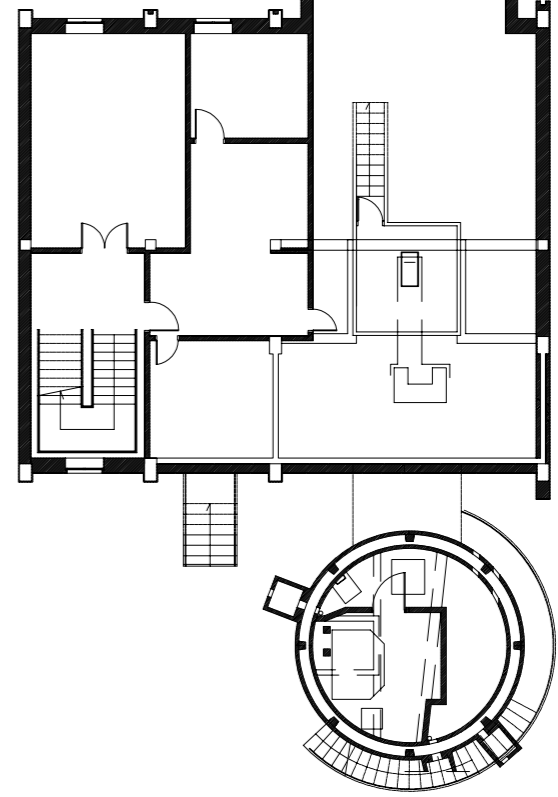
Plan du sous-sol N-1
